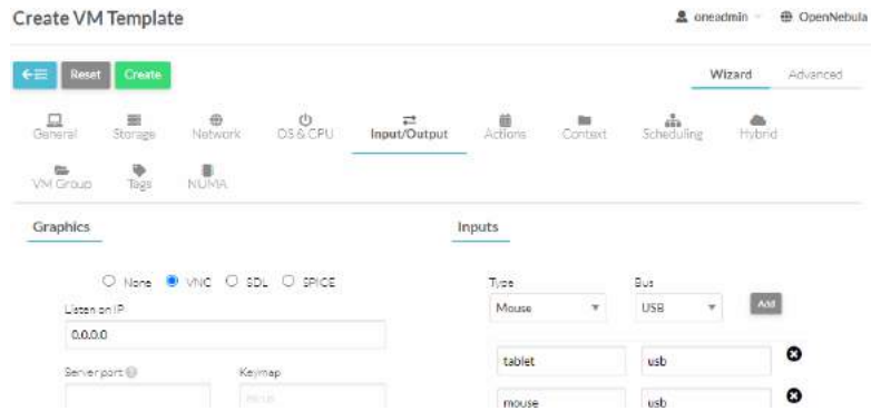
Figura 62. Gráficos y dispositivos de entrada para plantilla “servidorprueba”.
