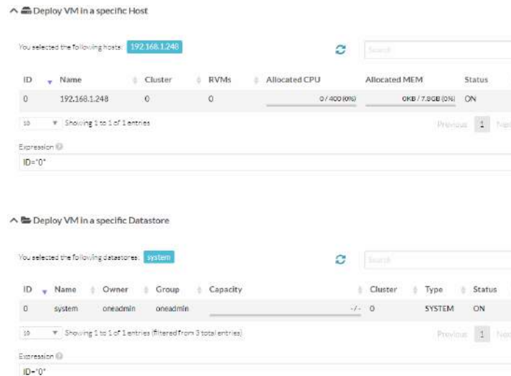
Figura 64. Selección de Host y Datastore específico para "servidorprueba".
