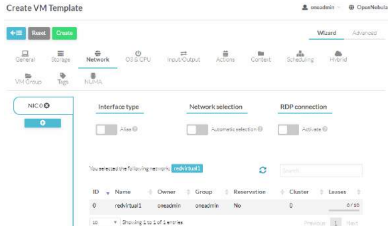
Figura 60. Selección de redvirtual1 para plantilla “servidorprueba”.
